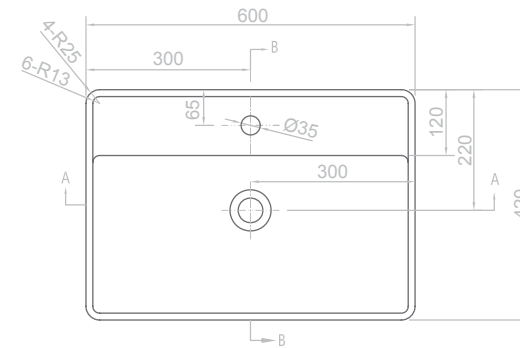
Lavatório de pé RECTANGULAR COM FURAÇÃO DE TORNEIRA
