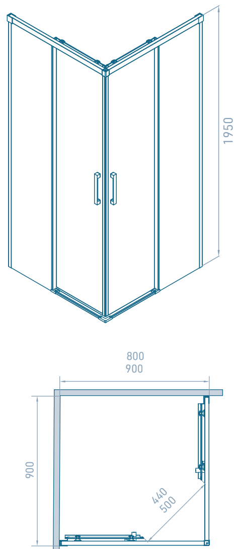
Desenho técnico
