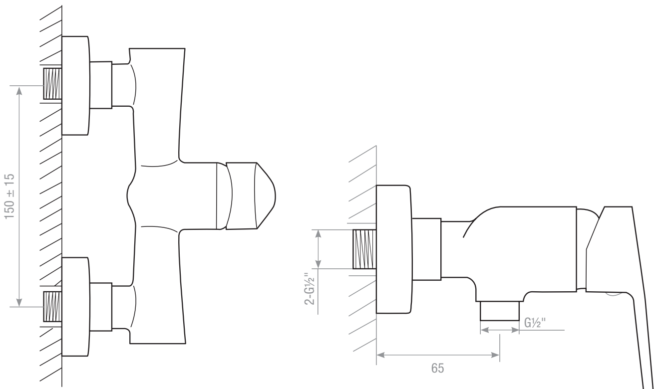
Desenho técnico (mm)
