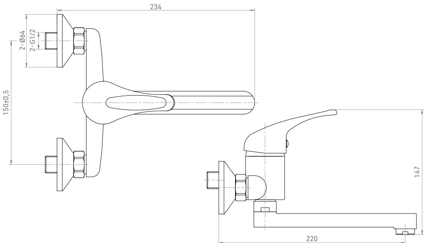
Desenho técnico
