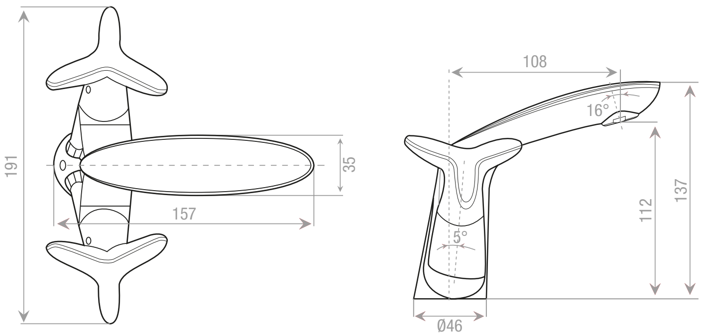
Desenho técnico (mm)
